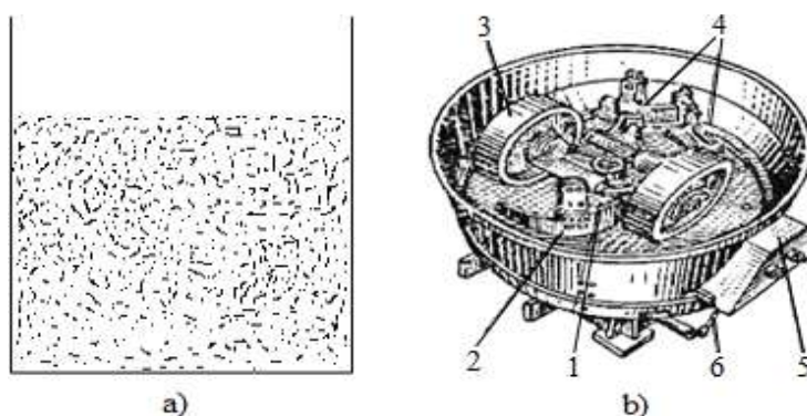
8.1-rasm. Qolip materiallari asosini tashkil etuvchi aralashmalar (a) va qolip materiallarini aralashtirib qorishtirish uchun mo'ljallangan qurilma mashinasi (b): 1-qurilmaning vertikal o'qi; 2-surgich; 3-g'ildirak; 4-surgich; 5-quti; 6-tortqi; 7-mahkamlangan holati.
