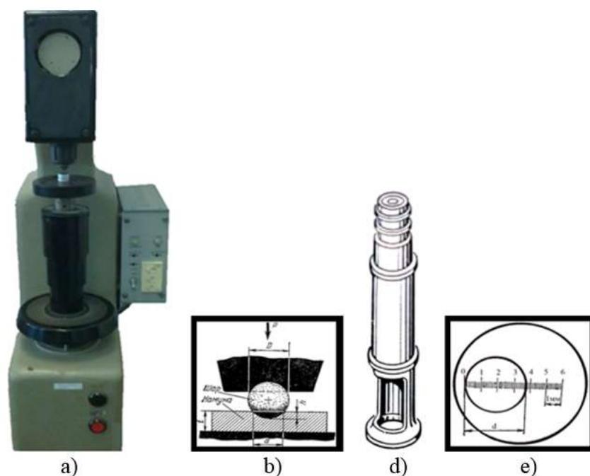
3.1-rasm. Brinel TB 5004 pribori umumiy ko‘rinishi (a), sinalayotgan materialga sharchani botirish jarayoni (b), botgan izni o‘lchash uchun maxsus optik lupa yoki mikroskop (d) va namuna yuzasida hosil bo‘lgan sharcha izining o‘lchangan holati (e).
