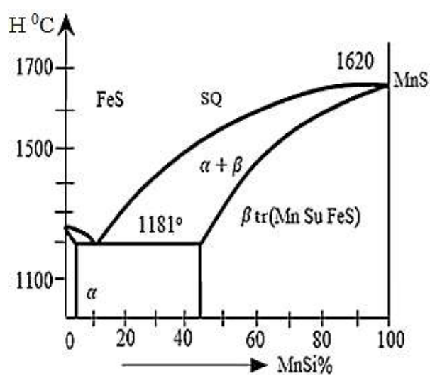
5-rasm. FeS–MnS sistemadagi qotishmalarning holat diagrammasi.
