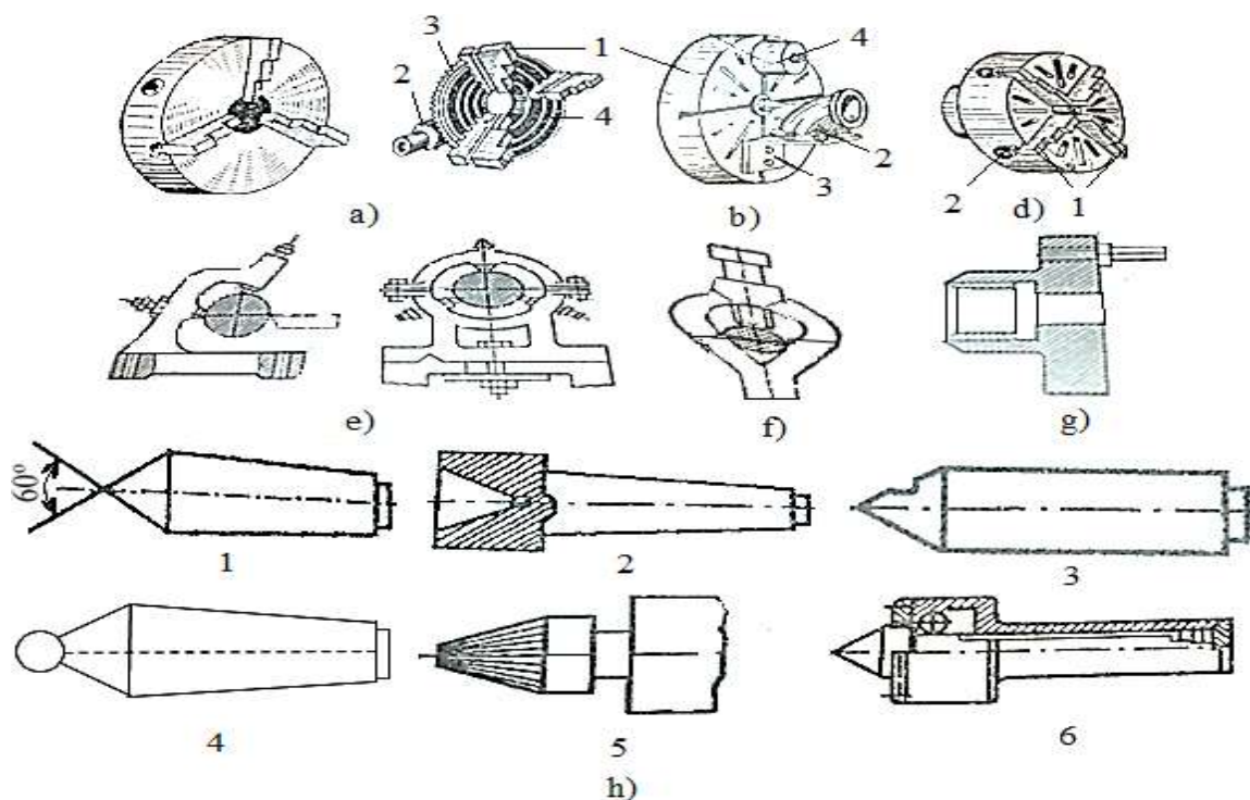
15.4-rasm. Tokarlik dastgohiga qo'shib beriladigan moslamalari: a -uch kulachokli patronlar; b -planshayba; 1-kulachoklar; 2-kichik konussimon shesternya; 3-katta konussimon shesternya; 4-spiral ariqchalar; d -to'rt kulachokli patron; 1-kulachoklar; 2-vint; e -lyunetlar; f -xomut; g -opravka; h -markazlar turi: 1-normal; 2-teskari; 3-kesik; 4-sharsimon; 5-tishli; 6-aylanuvchi markazlar ko'rinishlari.
