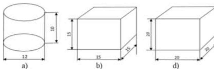
5.1-rasm. Qattqligi o'lchanadigan normal po'lat namunalarning o'lchamlari.
