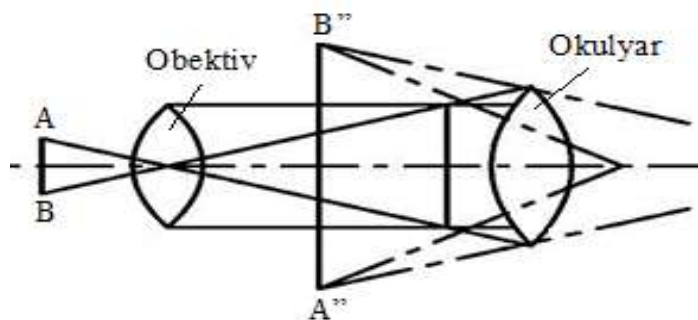
5.1-rasm. Namunadan qaytgan nurlarning linzalar sistemasidagi yo'nalishi.
