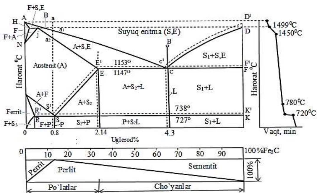
6.1-rasm. Temir-uglerod (temir-tsementit) holat diagrammasining po'lat bilan cho'yanga bo'lib ko'rsatilgan qismining tuzilishi.
