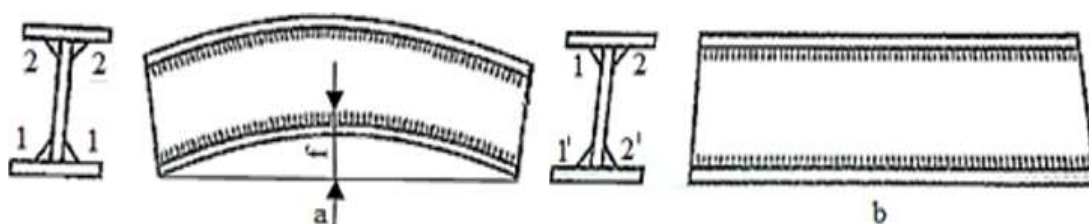
12.1-rasm. Metallarni noto'g'ri payvandlanish natijasida deformasiyalangan qo'shtavr balkasi (a) va to'g'ri payvandlangan qo'shtavr balkasi (b) ko'rinishlari.
