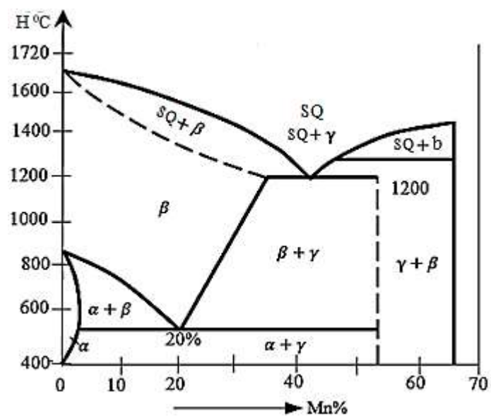
15-rasm. Ti–Mn sistemadagi qotishmalarning holat diagrammasi.
