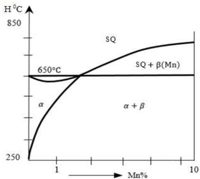
30-rasm. Mg–Mn sistemadagi qotishmalarning holat diagrammasi.
