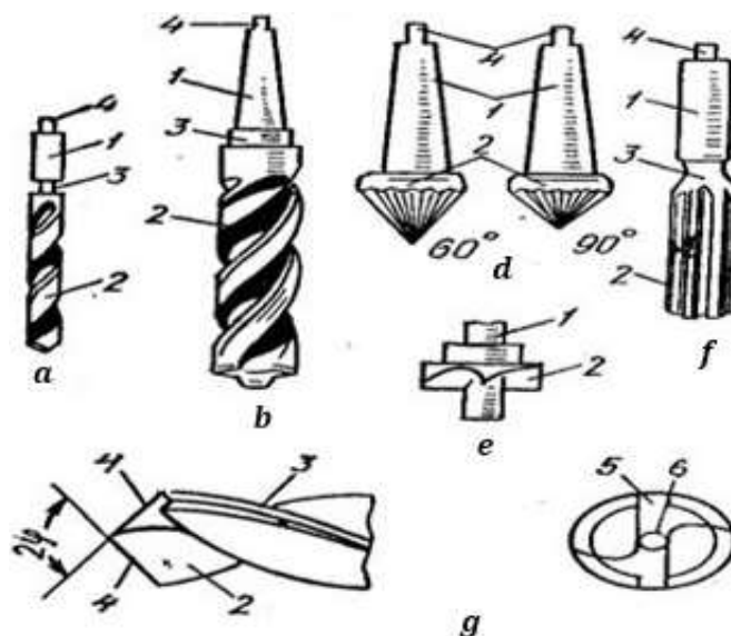
15.2-rasm. Dastgohga o'rnatiladigan parmalar turlari: a - spiral parma; b - slindrik zenker; d - zenkovkalar; e - sekovka; f - razvyortka; g - silindrik normal kesuvchi qism elementlari ko'rsatilgan: 1 - kesuvchi asosning tig'i; 2 - oldingi yuzasi; 3 - lentasi; 4 - yordamchi kesuvchi tig'i; 5 - ketingi yuzasi; 6 - ko'ndalang tig'i.
