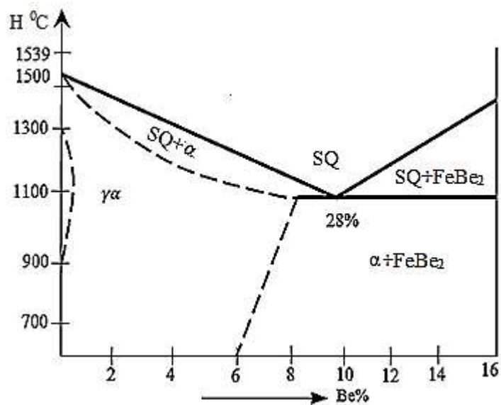
13-rasm. Fe–Be sistemadagi qotishmalarning holat diagrammasi.
