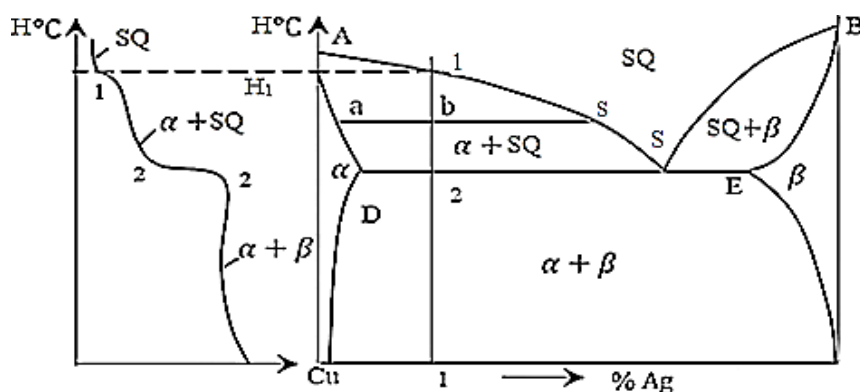
3.1-rasm. Cu-Ag holat diagrammasi va sovish egri chizig'i grafiting ko'rinishi.
