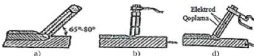
12.3-rasm. Metallarni dastaki payvandlashda ish unumini oshiruvchi usullar: a -metallni chuqurroq suyuqlantirib payvand chok birikma hosil qilish; b -elektrodlar tutami bilan payvandlash; d -uch fazali tok bilan payvandlash jarayonlari.
