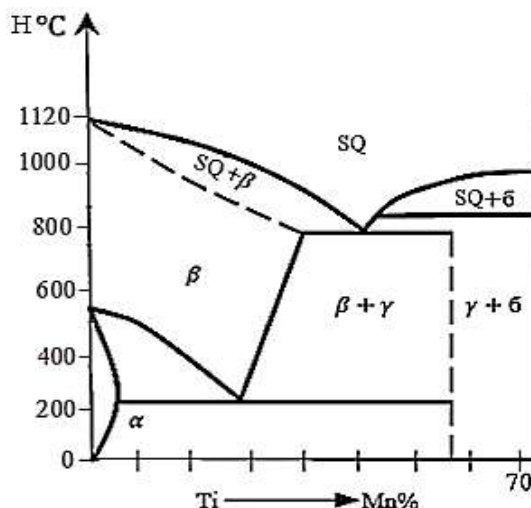
1-rasm. Ti–Mn cictemadagi qotishmalarning holat diagrammasi.
