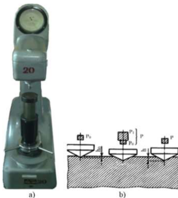
3.2-rasm. Qattiqlikni o'lchovchi Rokvel TK-2 priborining umumiy ko'rinishi (a) va po'lat namunani o'lchash ketma-ketliklari (b).
