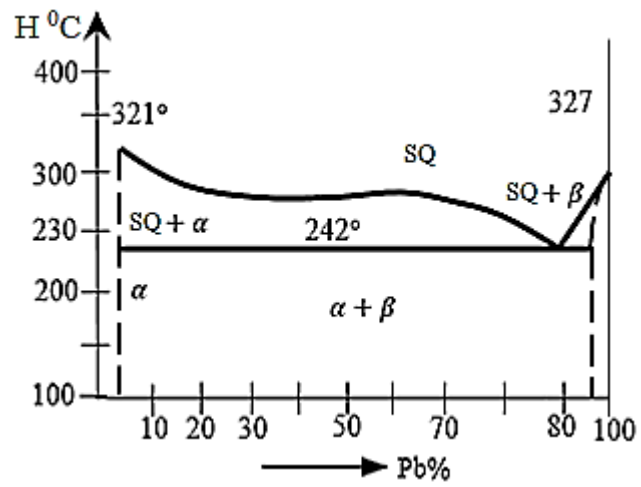
7-rasm. Cd-Pb sistemadagi qotishmalarning holat diagrammasi.
