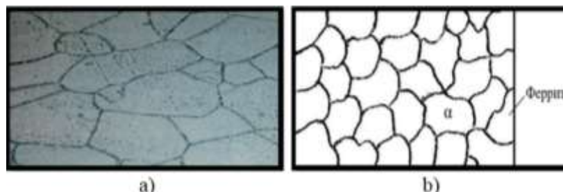
4.2-rasm. Texnika temirining mikrostrukturasi (a) X500 va sxemasi (b) ko'rinishlari.
