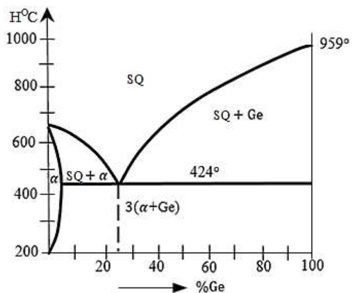
14-rasm. Al–Ge sistemadagi qotishmalarning holat diagrammasi.
