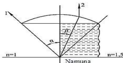
5.2-rasm. Imersiyali muhitning yorituvchanlik ta'siri.
