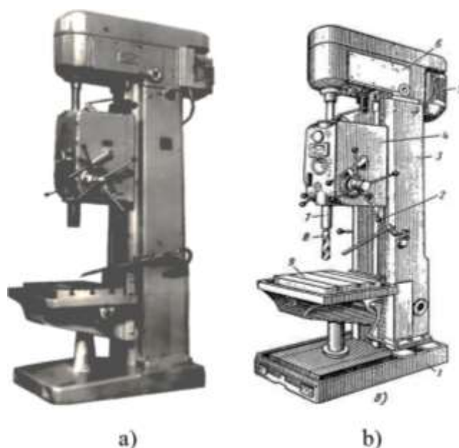
15.1-rasm. Parmalash dastgohining 2A150 modelini haqiqiy ko'rinishi (a) va sxematik tuzilishi (b): 1-poydevor plita; 2-qo'lda boshqarish richagi; 3-stanina; 4-surish qutisi; 5-elektro dvigateli; 6-tezliklar qutisi; 7-shpindeli; 8-parma; 9-stoli.
