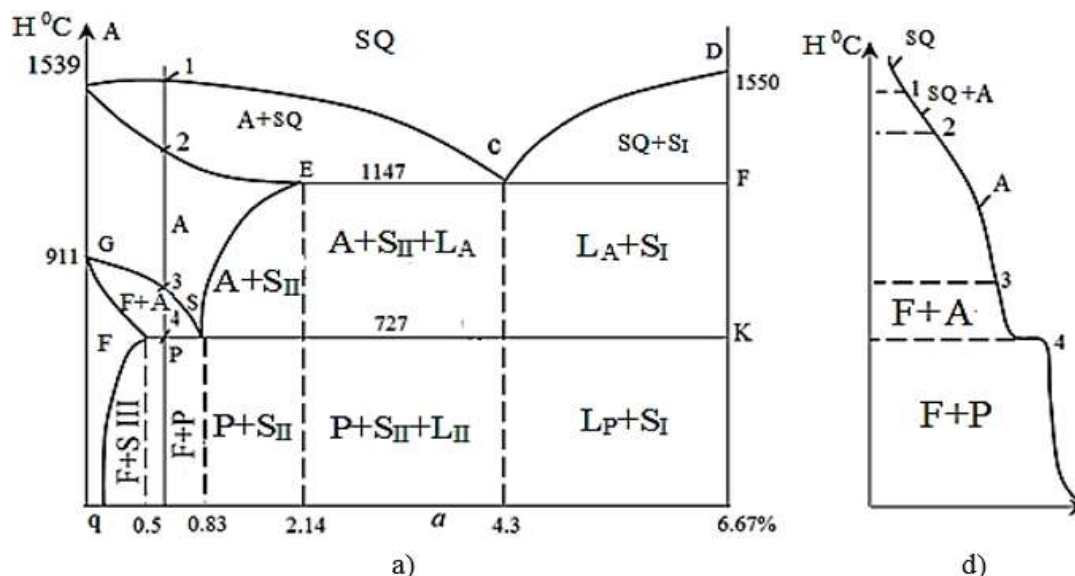
4.2-rasm. Qotishmalarning holat diagrammasi: a - Fe 3 C sistemalardagi qotishmalarning holat diagrammasi; b - S=0,5% qotishmaning sovish egri chizig'i.
