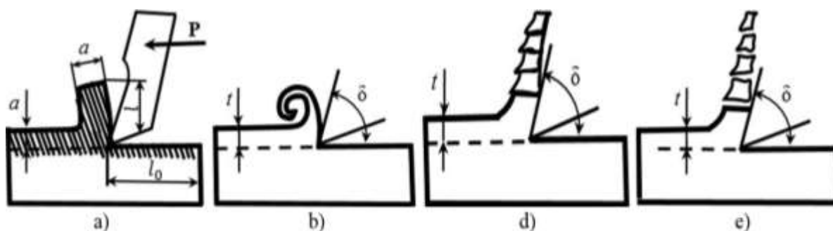
15.5-rasm. Metallarga kesib ishlov berish jarayonlari: a -metall qirindisining bo'ylama kirishuvi; b -tutash qirindi; d -yoriq qirindi; e -uvoq qirindi ajralib chiqish holatlari.
