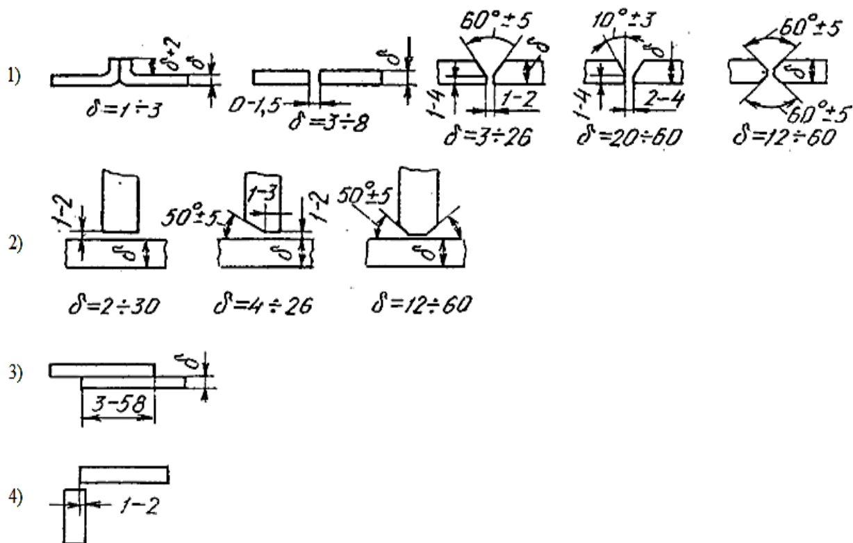
10.2-rasm. Metallarni dastaki payvandlash turlari: I-uchma-uch; II-tavroli; III-ustma-ust; IV-burchakli ko'rinishlari.
