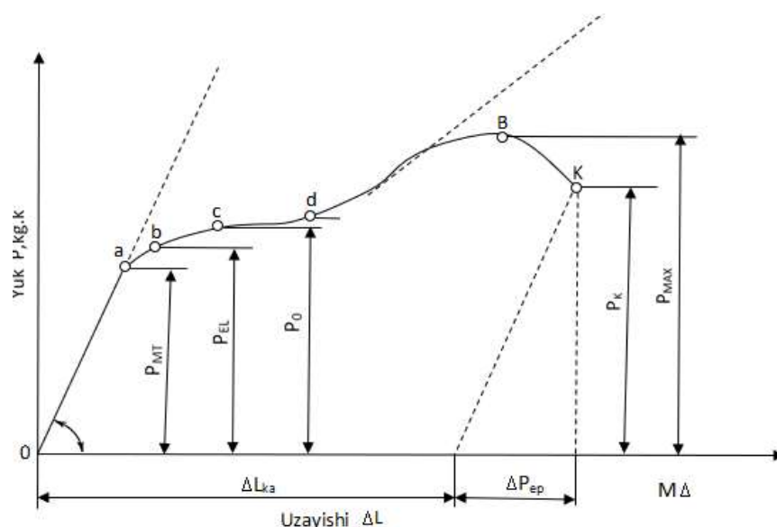
2.2-rasm. Kam uglerodli po'latdan tayyorlangan namunani sinashda deformatsiyalanish diagrammasining umumiy ko'rinishi.
