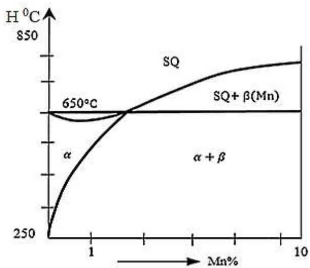
6-rasm. Mg–Mn sistemadagi qotishmalarning holat diagrammasi.
