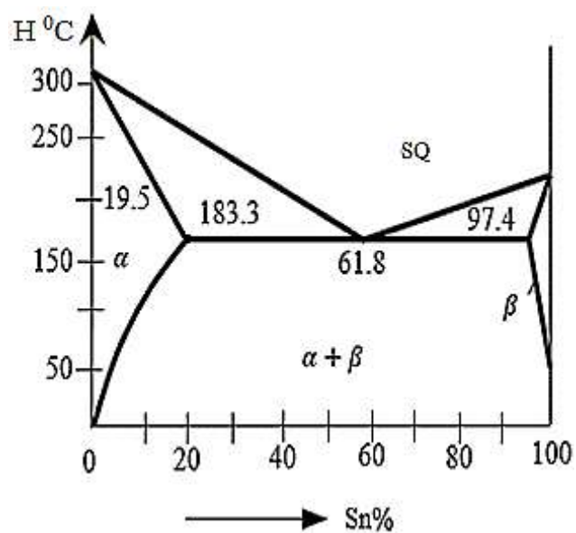
9-rasm. Pb–Sn sistemadagi qotishmalarning holat diagrammasi.
