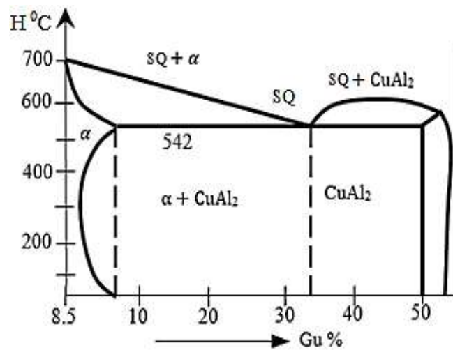
17-rasm. Al–Cu sistemadagi qotishmalarning holat diagrammasi.
