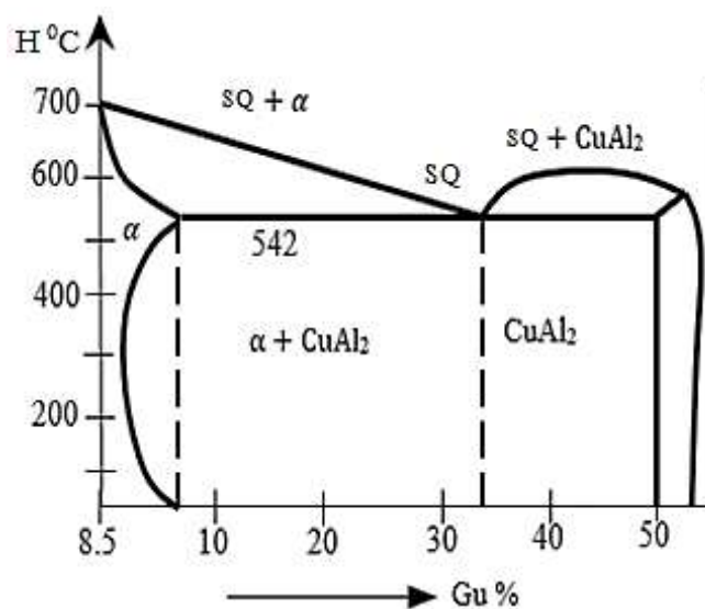
26-rasm. Al–Cu sistemadagi qotishmalarning holat diagrammasi.
