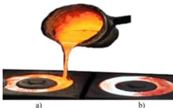
1.1-rasm. Yuqori haroratgacha qizdirib suyuqlantirilgan metallni formovka qilingan opokaga quyish holati (a) va quyilgan metallni sovish holati (b).
