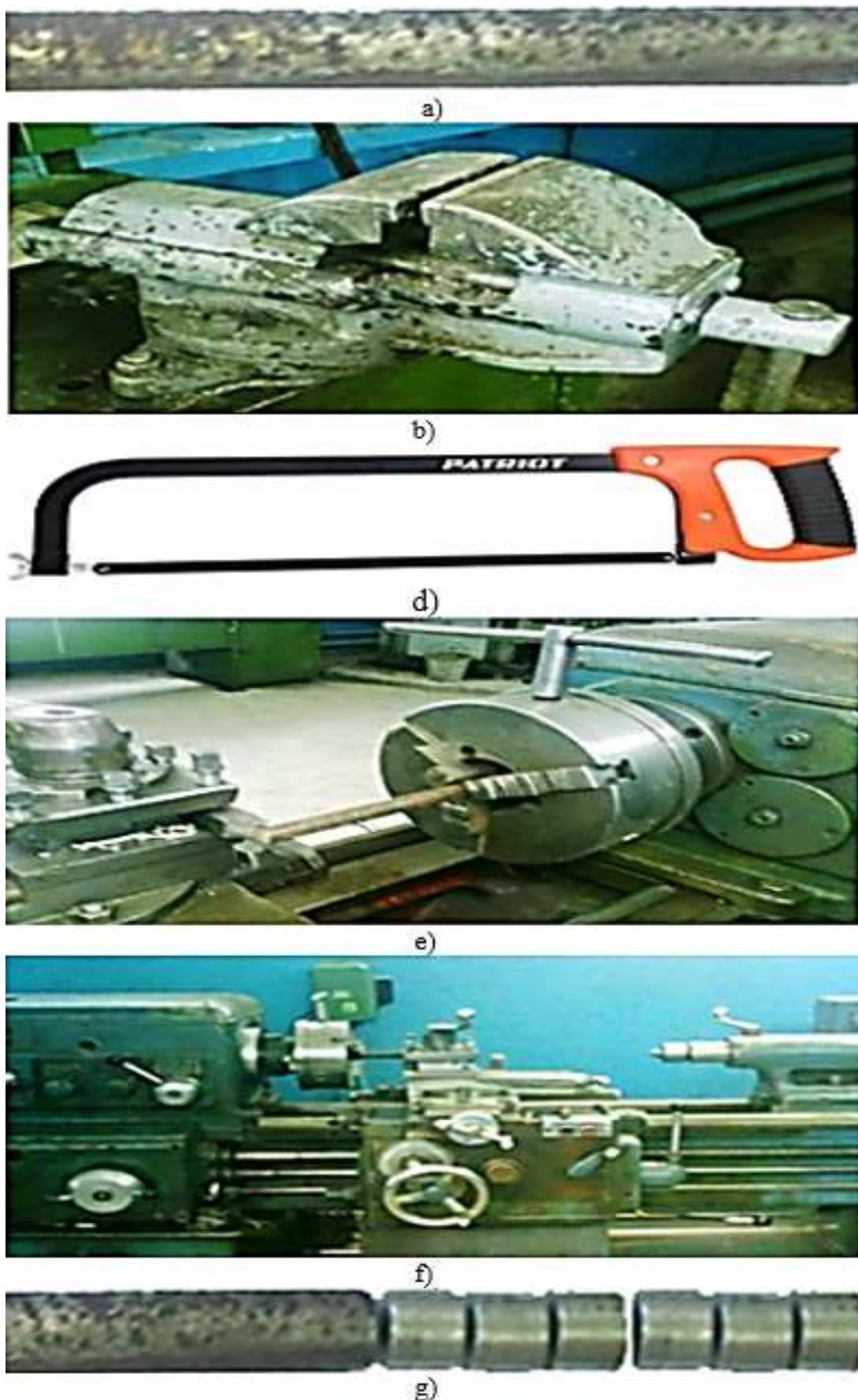
1.3-rasm. Po'lat prutok (a), tiska (b), qo'l arra (d), 1K62 tokarlik stanoki patroniga mahkamlab qotirilgan prutok (e), shu stanokda prutokni kesish vaqti (f) va bir necha bo'laklarga bo'lingan holati (g) ko'rinishlari.
