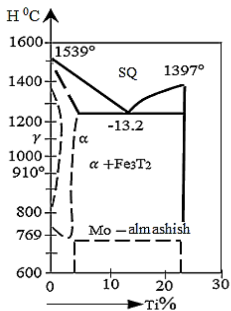
11-rasm. Fe–Ti sistemadagi qotishmalarning holat diagrammasi.
