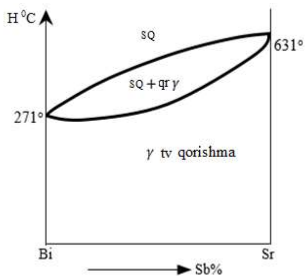
21-rasm. Bi–Sb sistemadagi qotishmalarning holat diagrammasi.
