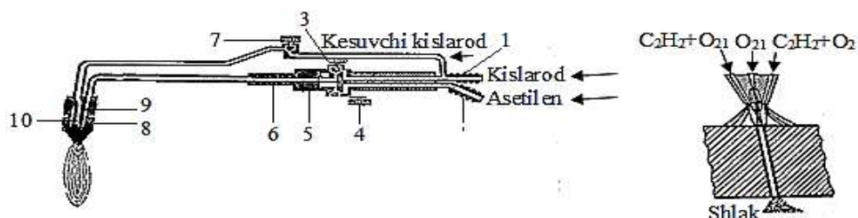
13.1-rasm. Universal UP xilidagi keskichning umumiy tuzilishi: 1,2-trubkalar; 3,4,7-ventillar; 5-injektor; 6-kamera; 8-mundshtuk; 9,10-asosiy teshiklar; 11-kislorod oqimidagi alanga.
