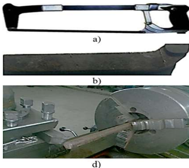
1.1-rasm. Makronamunalarni kesish jarayoni: a - metall keskich arra; b - maxsus keskich; d - tokarlik stanokida metall prutokni keskich bilan kesish vaqti.
