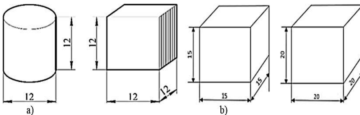
1.4-rasm. Po'lat prutok va kvadratdan maxsus o'lchamlarda kesilgan metall namunalarning umumiy ko'rinishlari: a -tsilindrik; b -to'g'ri burchakli.
