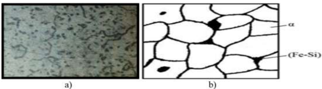
7.10-rasm. Duralyumin D16 qotishmasi: a -duralyuminning toblangan va tabiiy eskirtirilgan holatidagi mikrostrukturasi X200; b -sxemasi.
