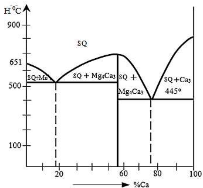
20-rasm. Mg–Ca sistemadagi qotishmalarning holat diagrammasi.
