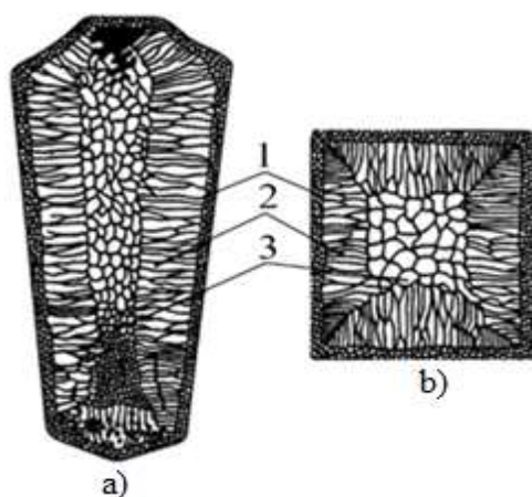
1.5-rasm. Quymakorlik usulida quyib olingan po'lat quymalarning (a,b) har xil zonalarga ajratilishi: 1-mayda donali zona; 2-uzunchoq kristallar zonasi; 3-teng o'qli kristallar zonasi tuzilishlari.
