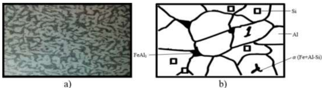
7.6-rasm. Alyuminiyning mikrostrukturasi (a) X200 va sxemasi (b).
