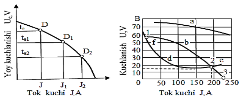
10.3-rasm. Metallarni payvandlash toki va elektr yoy manbalar xarakteristikasi: a -odatdagi tok manbainig xarakteristikasi; b -payvandlash tok manbainig xarateristikasi; d -yoyning xarakteristikasi; e -salt kuchlanish; f -yoyni barqaror yonishi grafigi.
