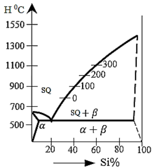
8-rasm. Al-Si sistemadagi qotishmalarning holat diagrammasi.
