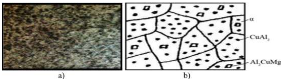
7.9-rasm. Duralyumin Д16 qotishmasi: a-duralyuminning yumshatilgan holatidagi mikrostrukturasi X200; b-sxemasi.
