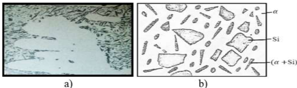
7.7-rasm. Oddiy siluminning mikrostrukturasi (a) X250 va sxemasi (b).
