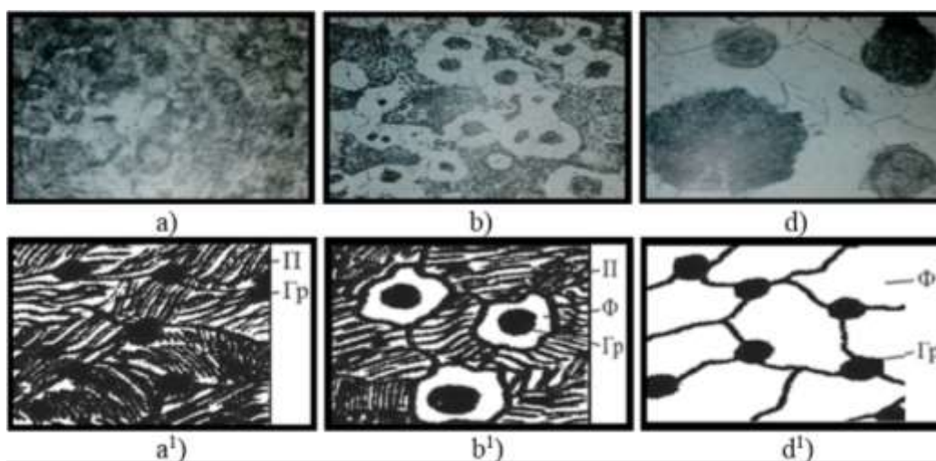
6.6-rasm. Juda puxta cho'yanlarning har xil shaklli mikrostrukturalari (a,b,d) X500 va ularning sxematik ko'rinishlari (a¹, b¹, d¹).
