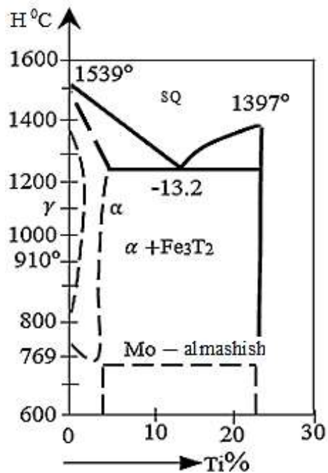
29-rasm. Fe–Ti sistemadagi qotishmalarning holat diagrammasi.
