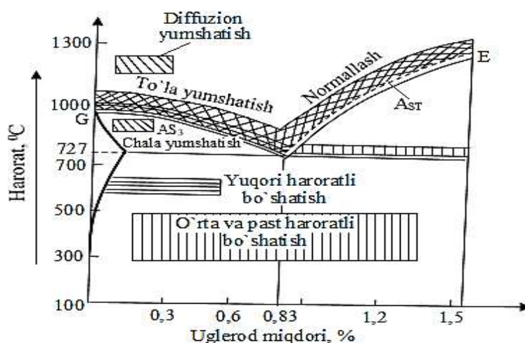
8.1-rasm. Po'latlarning uglerod miqdori o'zgarishi bo'yicha qizdirish haroratlarining borishi.
