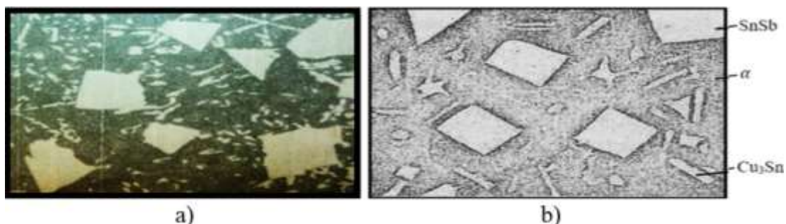
7.11-rasm. Qalayli B83 babbittni mikrostrukturasi ( a ) X100 va sxemasi ( b ).
