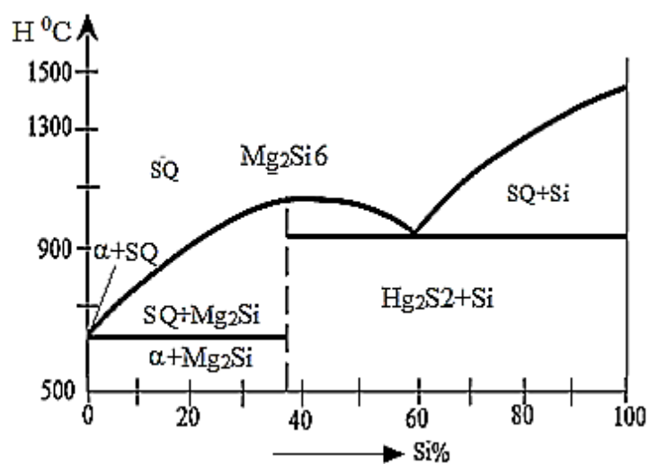
10-rasm. Mg–Si sistemadagi qotishmalarning holat diagrammasi.
