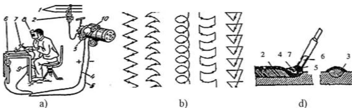
10.1-rasm. Metallarni dastaki payvandlash posti (a): 1-tok tarmog'i; 2-ulagich; 3-tok o'zgartirgich; 4,5-elektir simi; 6-zagotovka; 7-elektrod tutgich; 8-shit; 9-stol; 10-tok rostlagich; payvandlash sxemasi (b, d); 1-metall elektrod; 2-qoplama; 3-elektir yoy; 4-payvandlanuvchi metall; 5-shlak po'stloqining; 6-elektrod simi ko'rinishlari.
