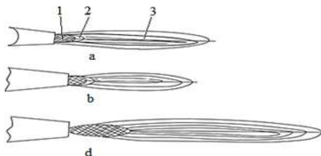
11.4-rasm. Metallarni payvandlashda gaz alangasining turlari: a -normal alanga; 1-o'zak qismi; 2-payvandlash zonasi; 3-mash'al zonasi; b -oksidlovchi alanga; d -uglerodlantiruvchi alanga ko'rinishlari.
