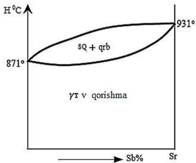
18-rasm. Bi–Sb sistemadagi qotishmalarning holat diagrammasi.
