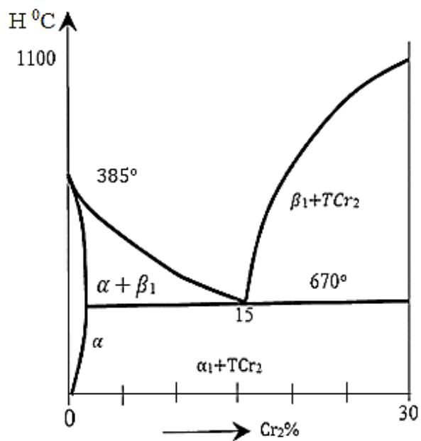
3-rasm. Ti–Cr sistemadagi qotishmalarning holat diagrammasi.
