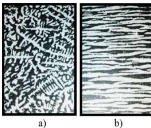
11.2-rasm. Metallarni bosim bilan ishlov berish haroratiga asosan quyma po'lat zagotovkali namunalarga sovuqlayin ishlov berilgan holatlari: a -ishlov berilmagan holatining mikrostrukturasi; b -ishlov berilgan holatining mikrostruktura tuzilishi. X100
