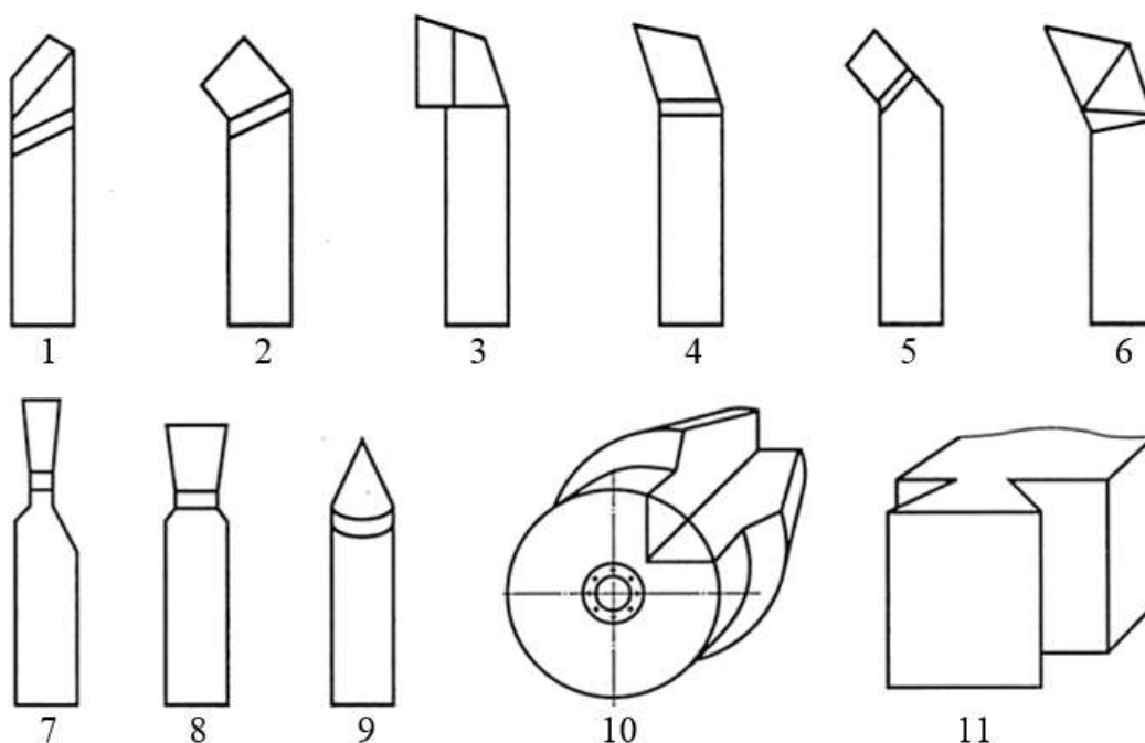
15.6-rasm. Tokarlik keskishlarining xillari: 1 -tog'ri o'tuvchi; 2 -burilib o'tuvchi; 3 -tayanch o'tuvchi; 4 -tiluvchi; 5,6 -mos ravishdagi ochiq va boshi berk teshiklarni yo'nib kengaytiruvchi; 7 -kesib tushiruvchi; 8 -ariqcha ochuvchi kanavkali; 9 -rezba kesuvchi; 10 -dumaloq shakldor; 11 -prizmatik shakldor.
