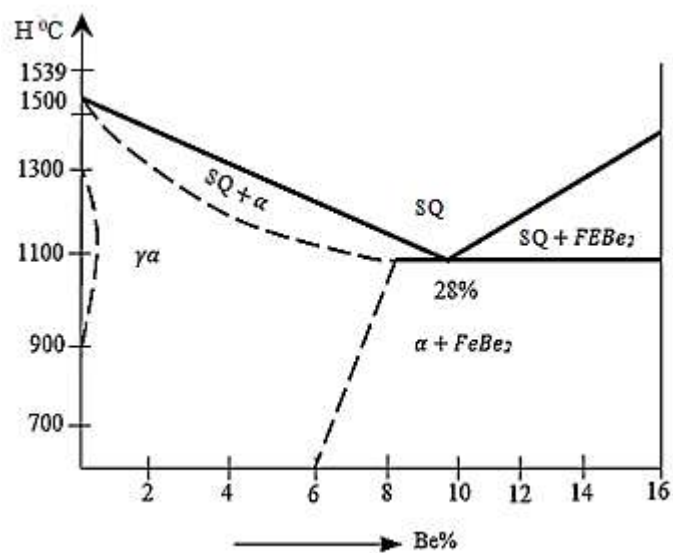
16-rasm. Fe–Be sistemadagi qotishmalarning holat diagrammasi.
