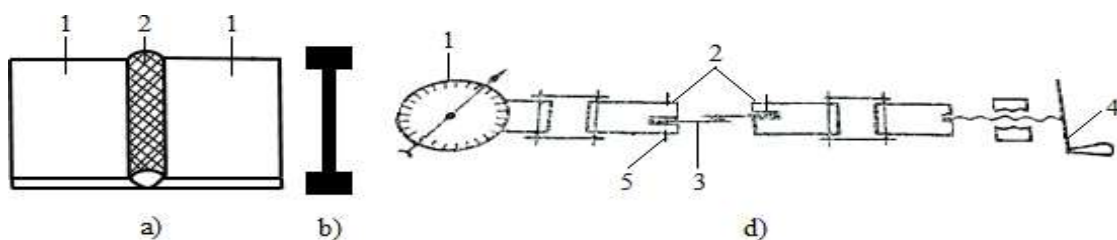
14.2-rasm. Namunada ajralmas birikma hosil bo'lgan joyi (a): 1,1-namuna, 2-payvand chok; cho'zilishga sinaladigan maxsus namuna (b) va kavsharlangan metall namunaning mustahkamligini cho'zilishga sinash mashinasining-priborining (d) umumiy ko'rinishlari.
