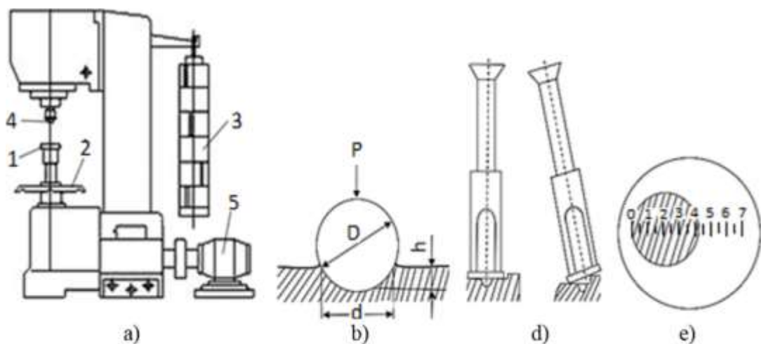
5.2-rasm. Brinel priborining sxemasi (a): 1-stol; 2-aylantirish rukoyatkasi; 3-yuklar; 4-po'lar shar; 5-pribor motori; sinalayotgan namunaga sharchani botishi (b); sharcha qoldirgan izning diametrini ko'rib aniqlash uchun lupa (d) va sharcha izining o'lchangan diametri (e).
