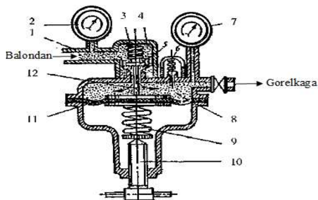
11.2-rasm. Ishlayotgan gaz reduktorining tuzilish va ishlash prinsipi: 1- reduktor korpusi; 2,7-manometr; 3,9-prujinalar; 4-yuqori bosimli kamera; 5-ehtiyot klapani; 8-quyi bosimli kamera; 10-vint; 11-membrana; 12-shtok ko'rinishlari.
