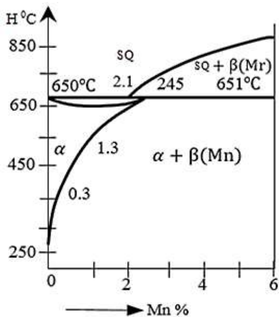
22-rasm. Mg–Mn sistemadagi qotishmalarning holat diagrammasi.
