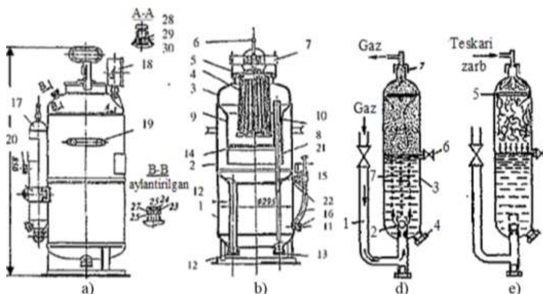
11.1-rasm. O'rta bosimda ishlaydigan ASM-1,25-3,0 markali atsetilen generatorining umumiy (a), bo'ylama kesimi (b), o'rta bosimda ishlovchi berk xilidagi suv qulfining normal ish davri (d) va teskari zarb davri (e): 1-yuvgich qismi; 2-gaz hosil qiluvchi qismi; 3-taglik; 4-korzina; 5-qopqoq; 6-vint; 7-richag; 8-trubka; 9-shaxta; 10-stakan; 11-nazorat krani; 12,13-chiqindilar chiqaradigan shtuserlar probkasi; 14-teshikli tarelka; 15-ehiyot klapani; 16-shlang; 17-suv qulfi; 18-manometr; 19-ko'tarish dastasi; 20-nazorat krani; 21-shtok; 22-shtuser; 23-gayka; 24-ehiyot to'r; 25,26-siquvchi halqalar; 27-membrana; 28-fibra prokladka; 29-rezina prokladka; 30-rezina prokladkalar oralig'idagi to'r ko'rinishlari.
