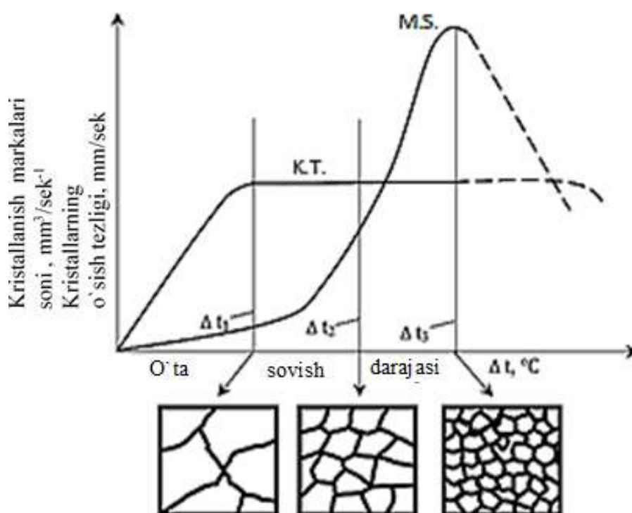
1.3-rasm. Metallardagi kristallanish markazlari soni va kristallarning chiziqli o'sish tezligining o'ta sovish darajasiga qarab o'zgarish grafigi.
