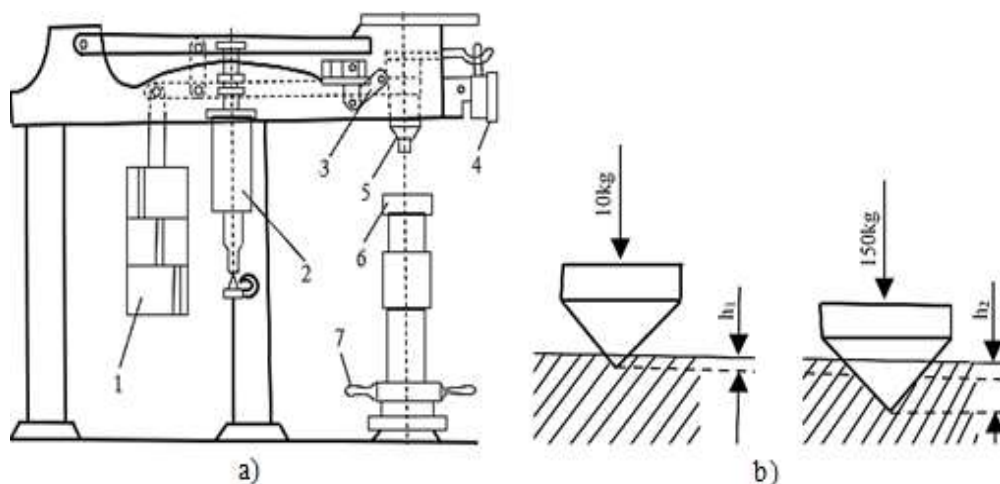
5.3-rasm. Namunalar qattqligini o'lchovchi Rokvel TK-2 priborining sxematik ko'rinishi (a) va namunaga har xil yuklar ta'sirida uchlik botgan izlar chuqurliklari (b); h_1 va h_2 olmos uchlik botgan izlar diametri.
