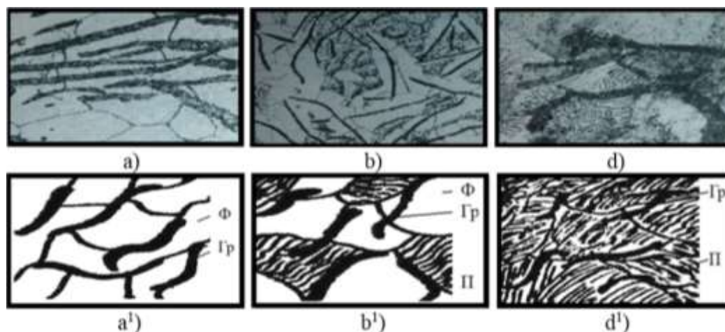
6.3-rasm. Kulrang cho‘yanlarning har xil shaklli mikrostrukturalari (a,b,d) X500 va ularning sxematik ko‘rinishlari (a 1 , b 1 , d 1 ).
