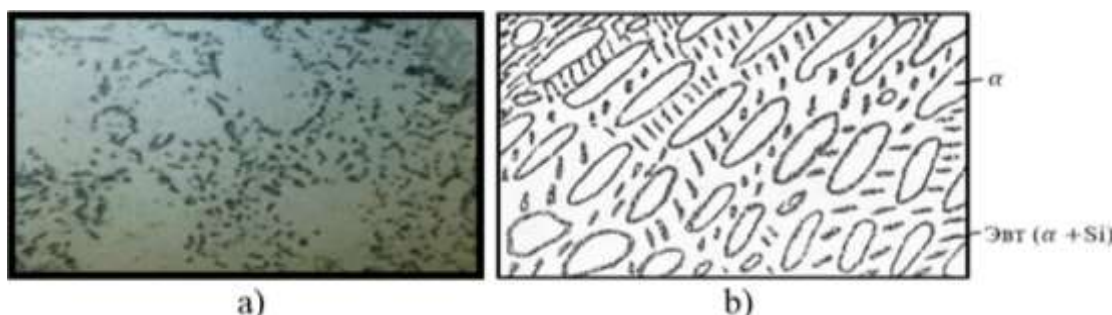
7.8-rasm. Modifikatsiyalangan siluminni mikrostrukturasi (a) X250 va sxemasi (b).
