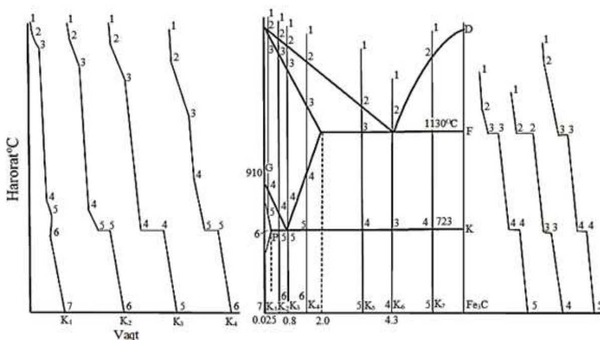
6.2-rasm. Metall va qotishmalarni qizdirish va sovutishda hosil bo'lgan grafiklarning ko'rinishlari.
