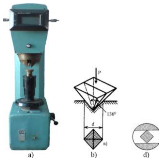
5.4-rasm. Vickers priborining umumiy ko'rinishi (a), po'lat namuna yuza qatlamidagi qalinlikni olmos piramida bilan o'lchayotganda hosil bo'lgan iz diagonali (b) va shu namuna tashqi yuzasida olmos piramida bosimida olingan iz o'lchamining (d) sxematik tuzilishlari.
