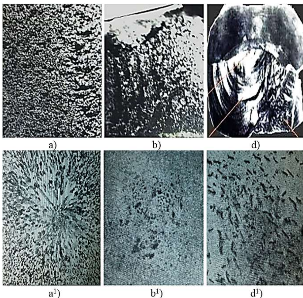
2.2-rasm. Mashina detallaridagi qovushqoq ( a ), mo'rt ( b ) va toliqish oqibatida sinish ( d ) hamda quyma po'lat strukturasi ( a 1 ), g'ovaklar ( b 1 ) va yoriqlar ( d 1 ) ko'rinishlari. X200
