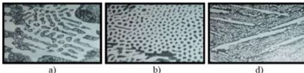
6.2-rasm. Oq cho‘yanning evtektikagacha (a), evtektikali (b) va evtektikadan keyingi (d) mikrostrukturalari. X500
