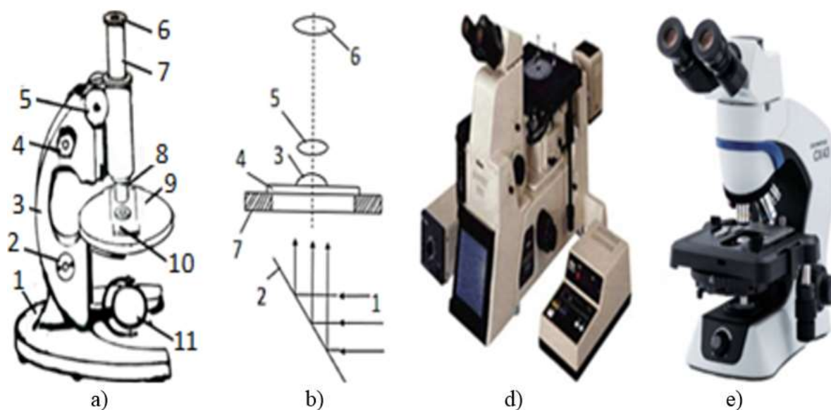
1.6-rasm. Biologik mikroskopning umumiy tuzilishi (a), optik sxemasi (b) va haqiqiy avvalgi (d) va hozirgi yangi zamonaviy (e) ko'rinishlari: 1-taglik plitasi; 2-sharnir; 3-kolonna; 4-mikrovint; 5-vint; 6-okulyar; 7-tubus; 8-ob'ektiv; 9-stol; 10-sirlanmagan oyna va ustida tuz eritmasi; 11-nur yo'nalishini rostlovchi sirlangan oyna; optik sxemasi bo'yicha 1-yorug'lik nurini yo'nalishi; 2-sirlangan oyna; 3-tuz eritmalarining tomchisi; 4-sirlanmagan oyna; 5-ob'ektiv; 6-okulyar; 7-mikroskop stoli.
