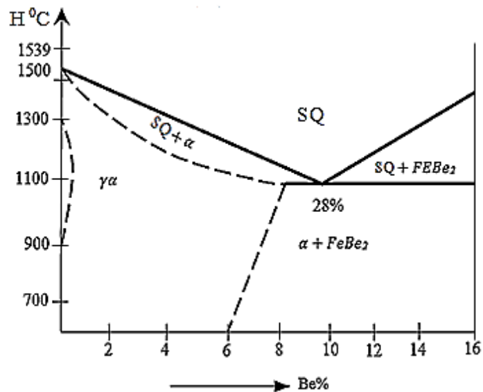
28-rasm. Fe–Be sistemadagi qotishmalarning holat diagrammasi.
