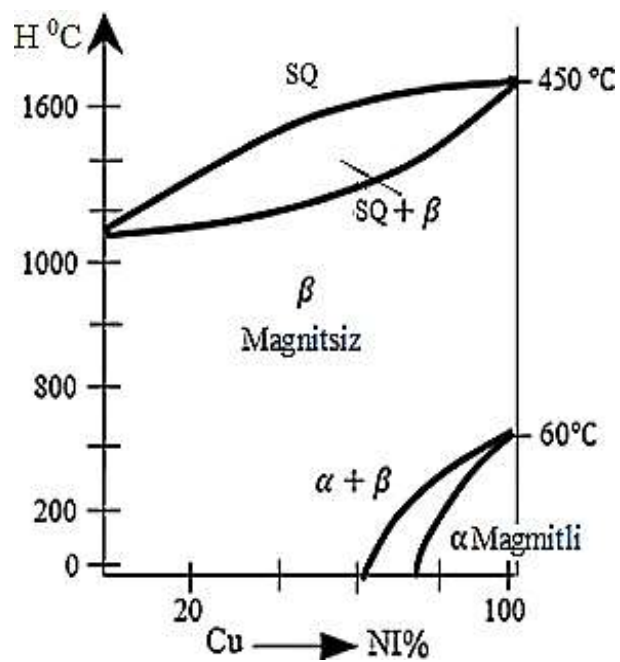
4-rasm. Cu–Ni sistemadagi qotishmalarning holat diagrammasi.
