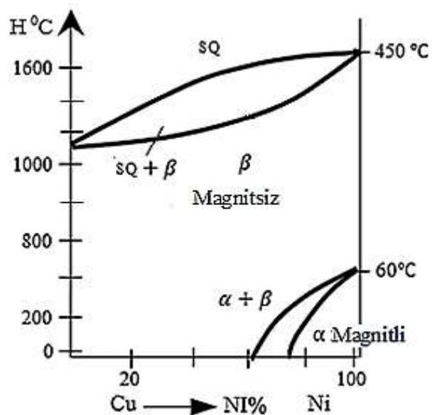
23-rasm. Cu–Ni sistemadagi qotishmalarning holat diagrammasi.
