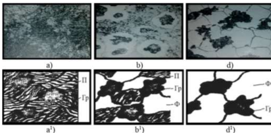
Ris.6.5. Bolg'alanuvchi cho'yanlarning har xil shaklli mikrostrukturalari (a,b,d) X500 va ularning sxematik ko'rinishlari (a', b', d').
