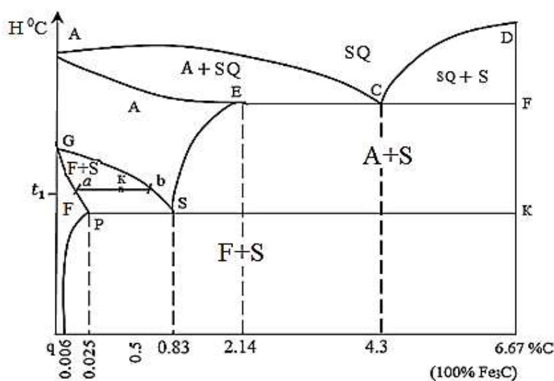
4.1-rasm. Fe– Fe_3C sistemadagi qotishmalarning fazalari ko'rsatiladigan holat diagrammasining ko'rinishi.
