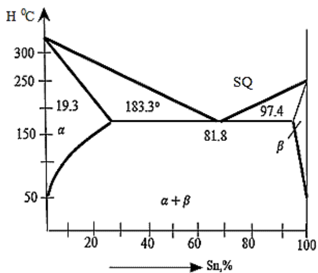
12-rasm. Pb–Sn sistemadagi qotishmalarning holat diagrammasi.
