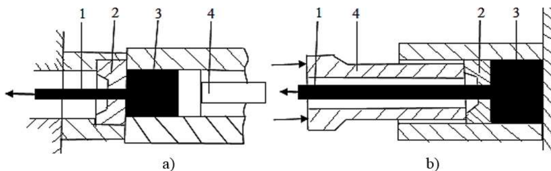
11.4-rasm. Po'lat prutokni to'g'ri presslash (a) va teskari presslash (b) usullari: 1-tayyor prutok; 2-matritsa; 3-zagotovka; 4-puanson.
