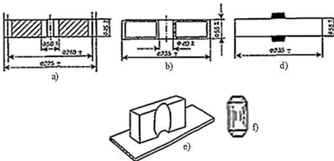
8.2-rasm. Quymakorlik usuli yordamida qolip yasash uchun kerakli materiallar: a -detal chizmasi; b -quyma zagotovka chizmasi; d -yog'och model; e -sterjen yashigi; f -sterjenning o'zini ko'rinishlari.
