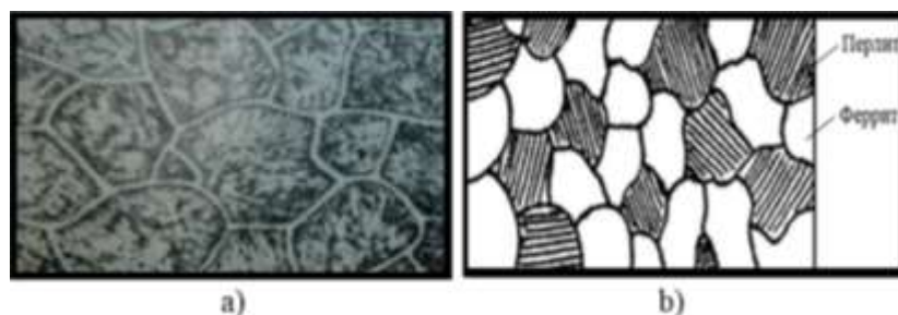
4.3-rasm. Evtektoidgacha bo'lgan po'latning mikrostrukturasi (a) X500 va sxemasi (b) ko'rinishlari.
