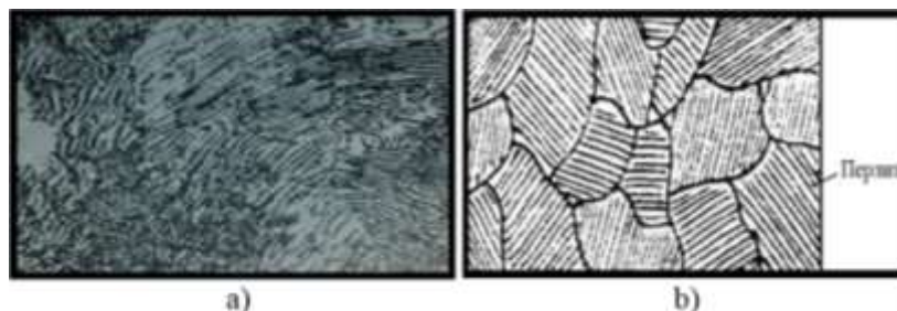
4.4-rasm. Evtektoidli po'latning mikrostrukturasi (a) X500 va sxemasi (b) ko'rinishlari.
