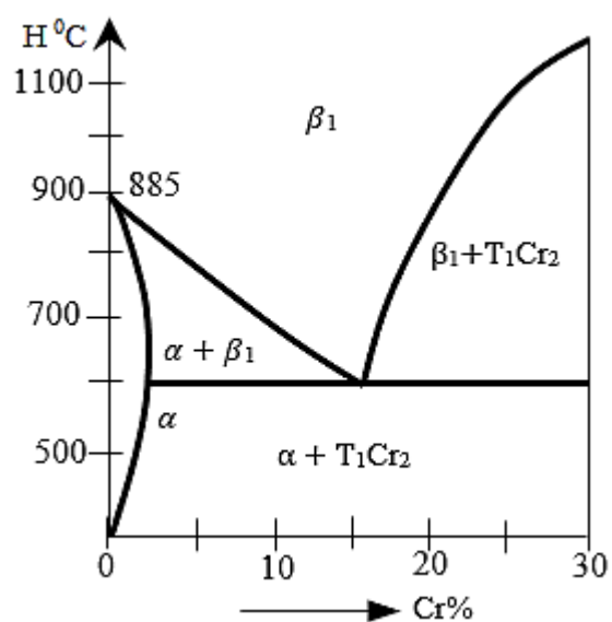
25-rasm. Ti–Cr sistemadagi qotishmalarning holat diagrammasi.
